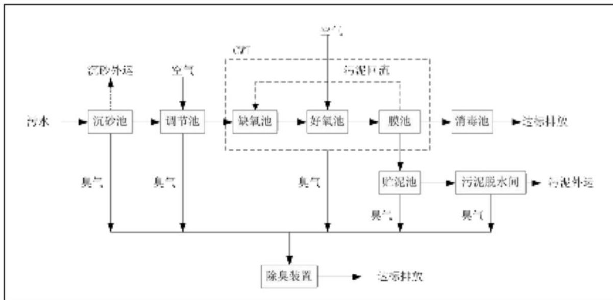
图 4-2 阳春市三甲镇生活污水处理厂处理工艺流程图
