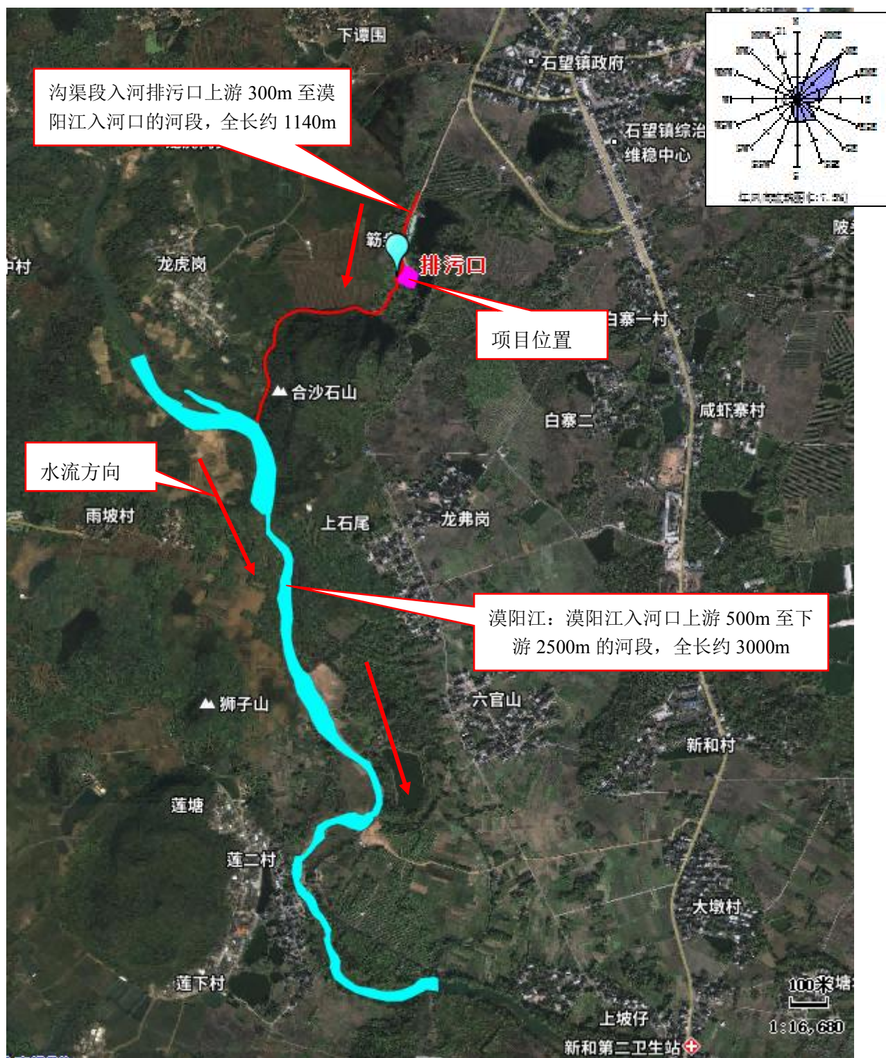
图 1.3-2 项目论证范围图
