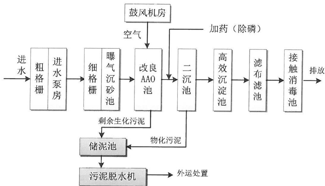
图2.2-1 阳春市马水镇生活污水处理厂处理工艺流程图
