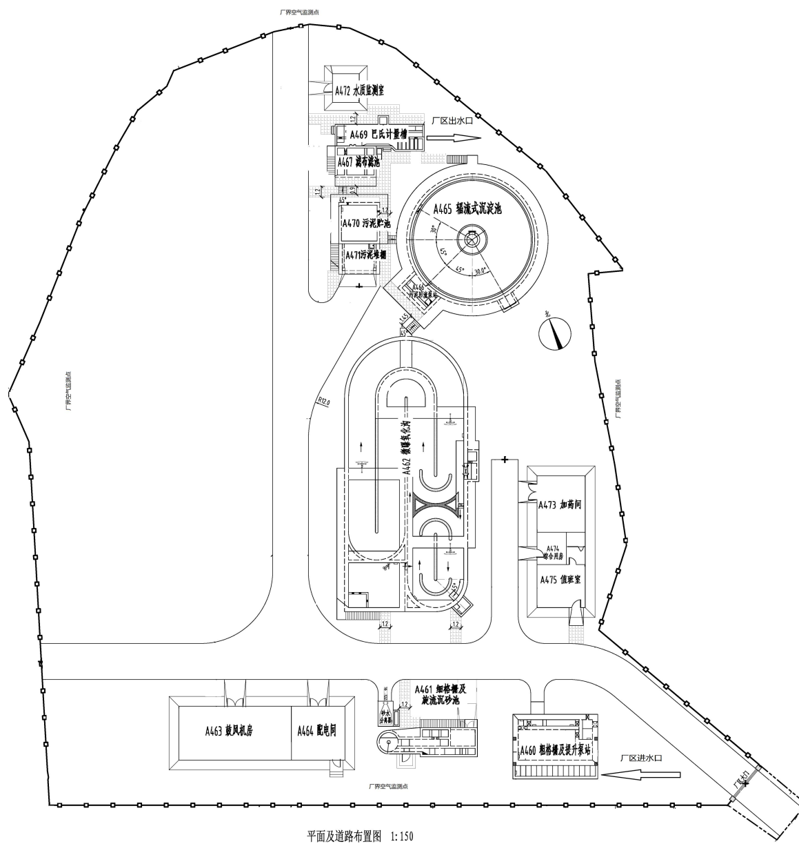
附图 6 项目总平面布置图
