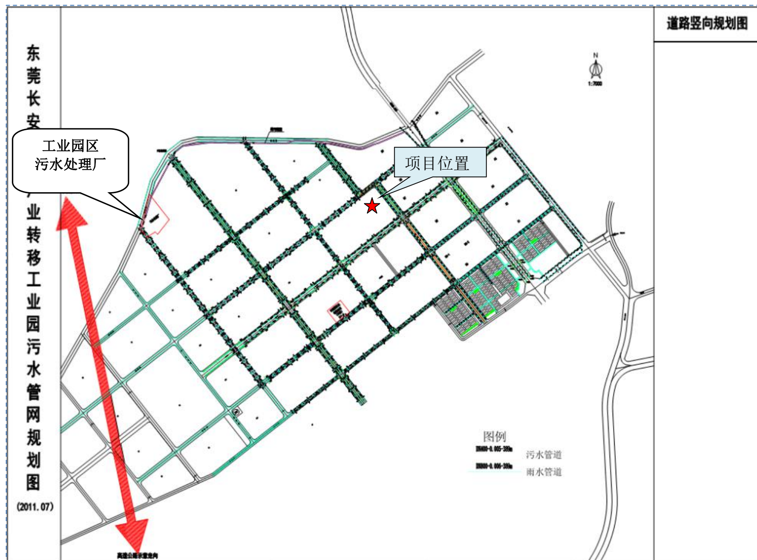
附图 10 工业园区污水管网分布图
